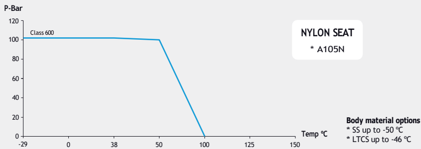
Fig. 560 (Class 600)
