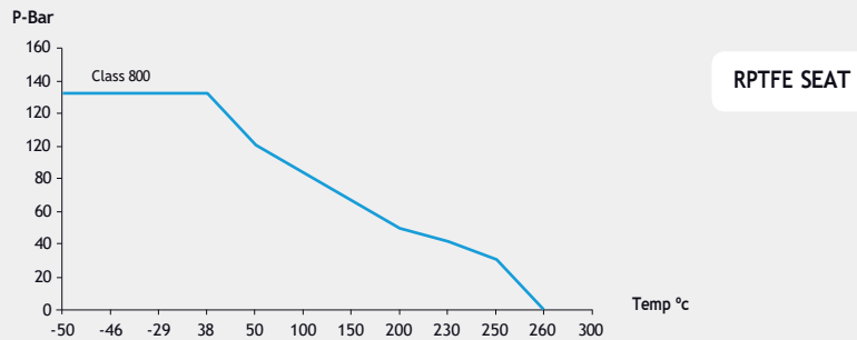
Fig. 411N (Class 800)
