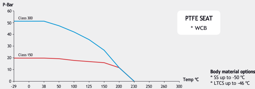
Fig. 1515 (Class 150)
