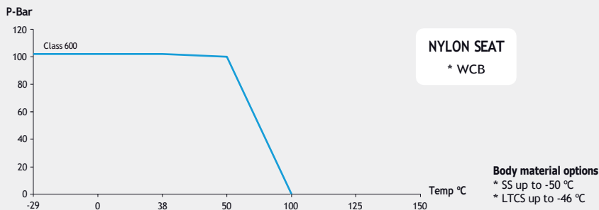
Fig. 660 (Class 600)
