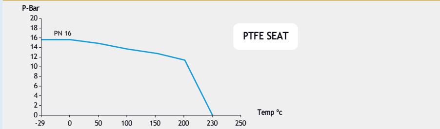
Fig. 512 (PN 16)
