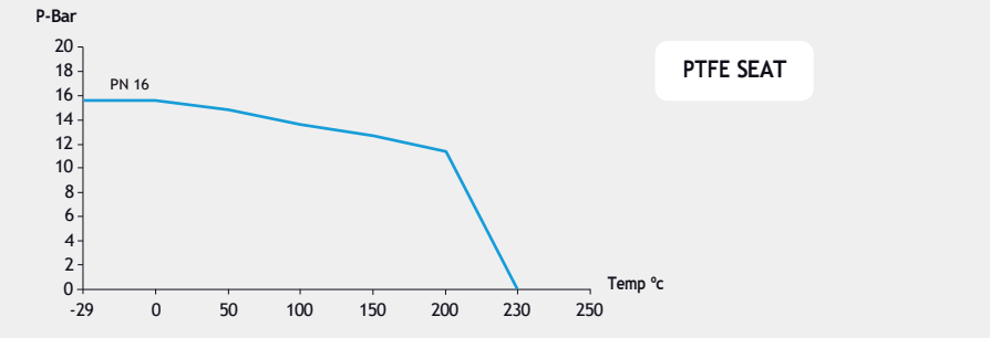
Fig. 916 (PN 16)
