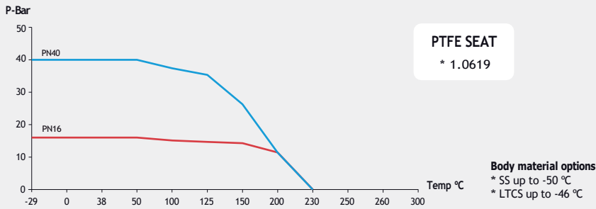
Fig. 1516 (PN 16)
